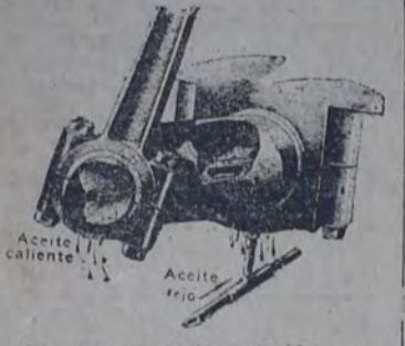
Fig. 1. — La cabeza de biela sufre por el hecho de que el aceite que ella recibe ha sido previamente calentado en los cojinetes de bancada del motor.
