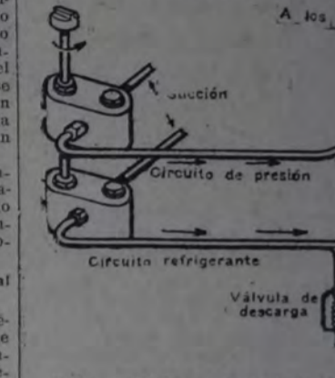
Fig. 7. — El último sistema R. Schneider está provisto de dos bombas independientes, una para alimentar los cojinetes y otra para mantener la circulación a través del radiador, el que puede anularse por medio de una llave de paso.
