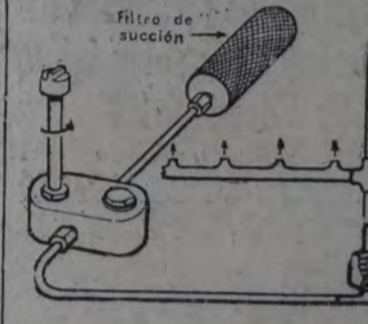
Fig. 6. — El sistema Peugeot es notable por la provisión de una válvula de descarga en paralelo con el radiador de aceite, a través de la cual el lubricante escapa cuando el motor arranca en fría.
