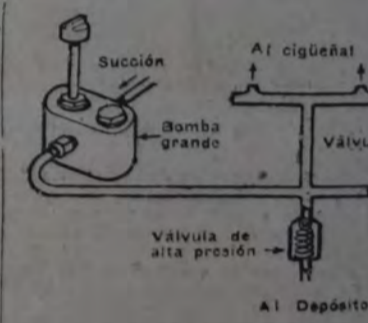
Fig. 8. — En este esquema una cantidad de aceite mandado por la bomba se descarga por medio de una válvula a un radiador, de donde pasa para ir de nuevo al depósito.
