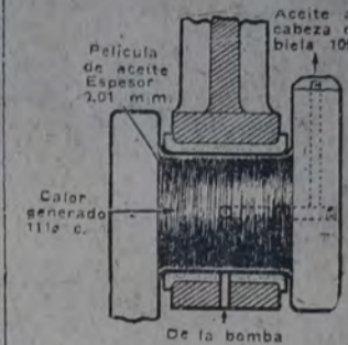
Fig. 4. — Un cigüeñal puede fácilmente alcanzar una temperatura de 95 grados centígrados, de modo que la película de aceite se calienta por conducción y fricción.
